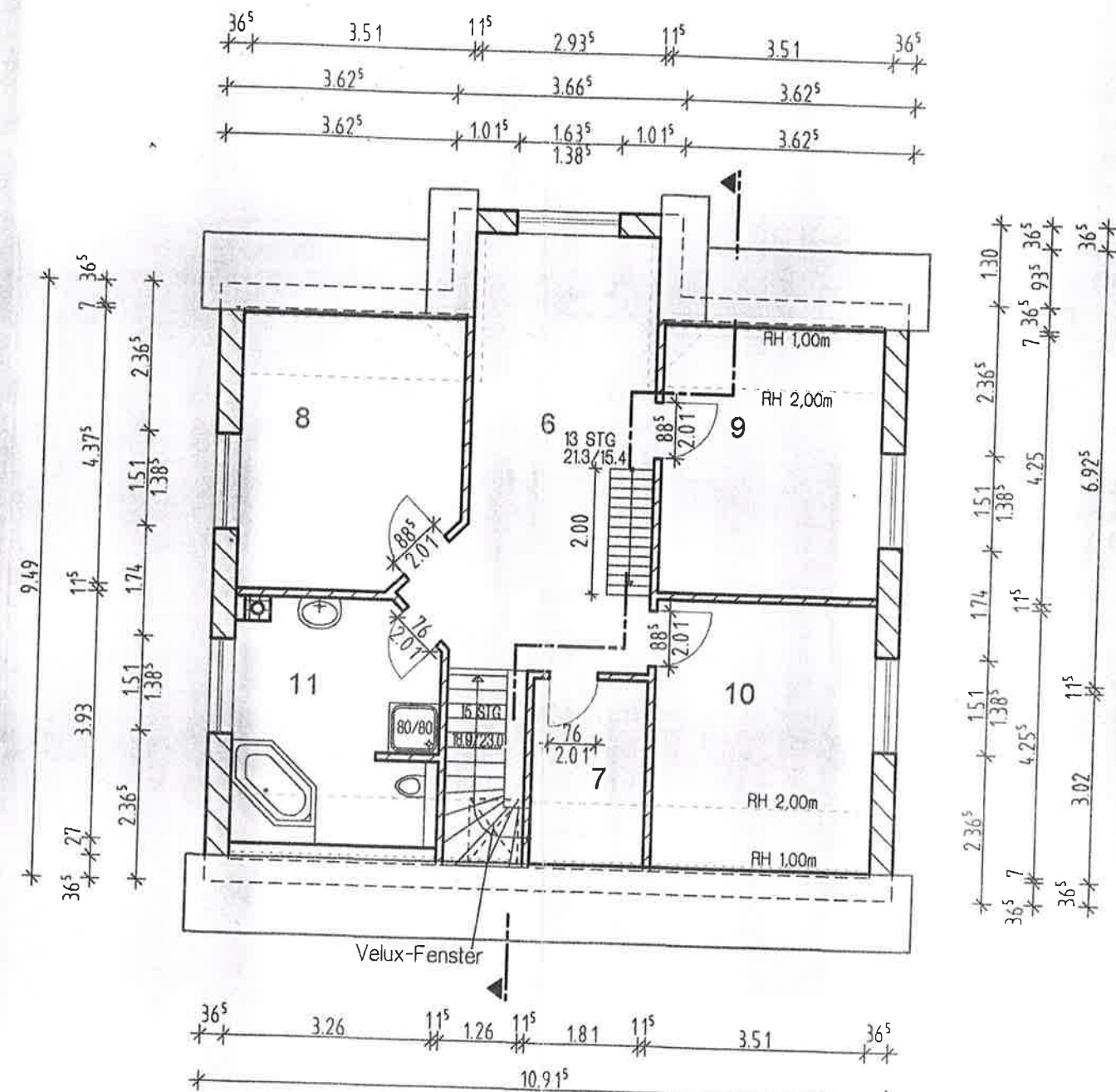
Grundriss DG
