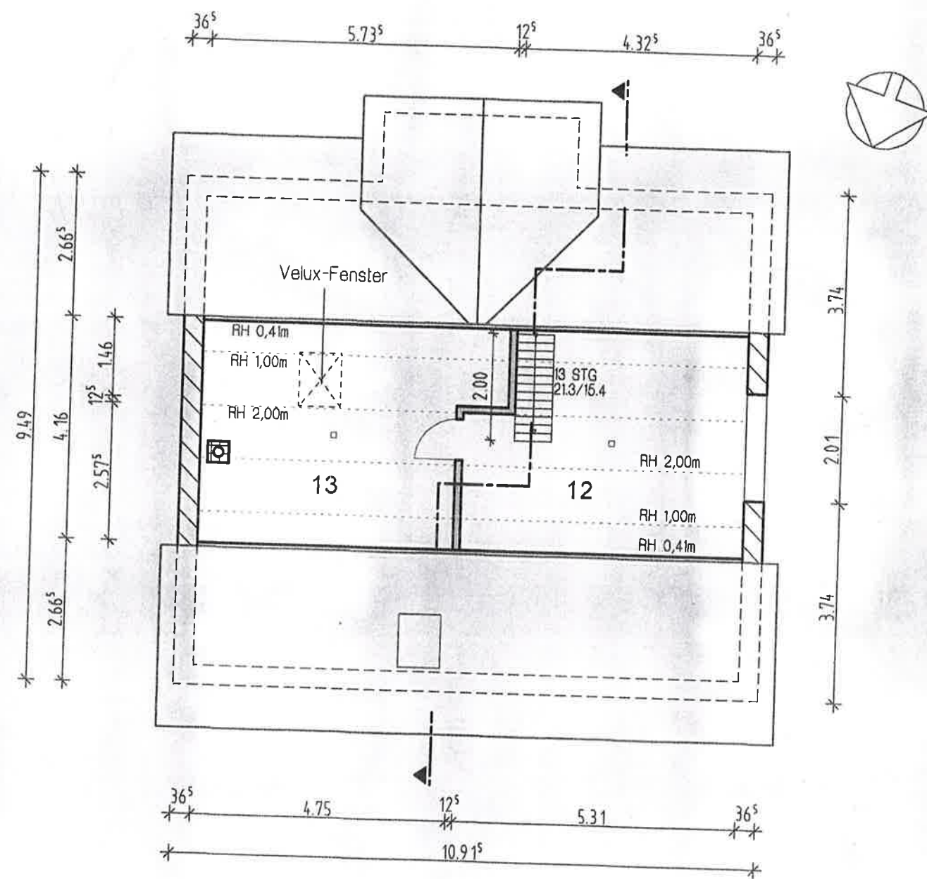
Grundriss Spitzboden
